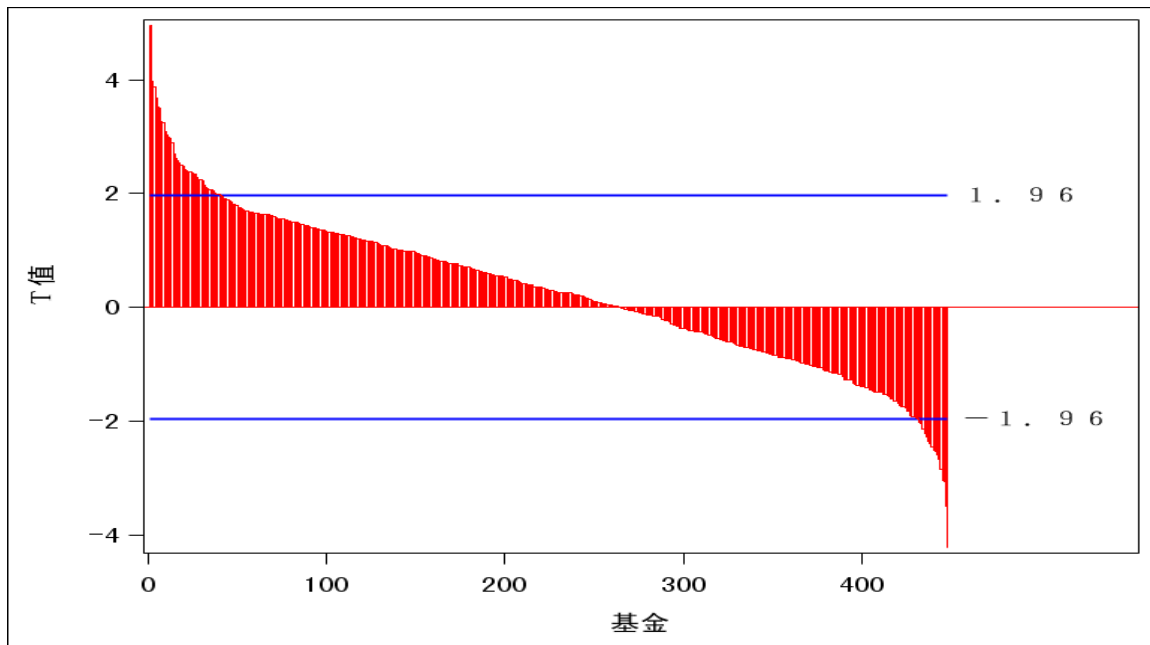
图 3 T-M 模型中 \gamma 的 t 值(从高到低)
